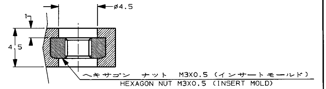
SECT A-A
