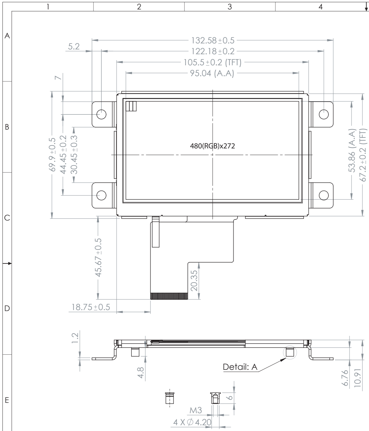
Detail: A 1:1
